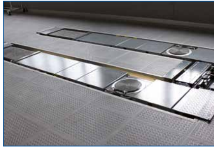
DUO CM im Streifenfundament (Ausstattung für Fahrwerksvermessung).
